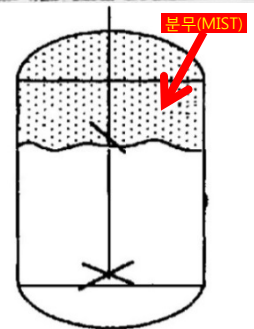
그림 2: 교반기로 인해 매우 작은 가연성 액적분무가 형성
